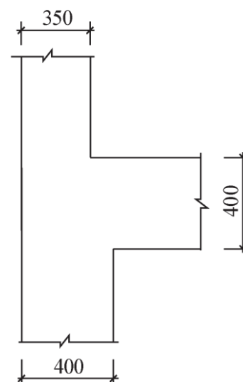
Hình 2. Nút khung
