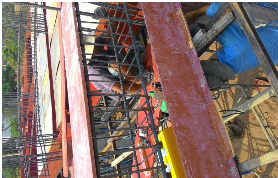
Hình 2.5: Thực hiện cốp pha đầm
